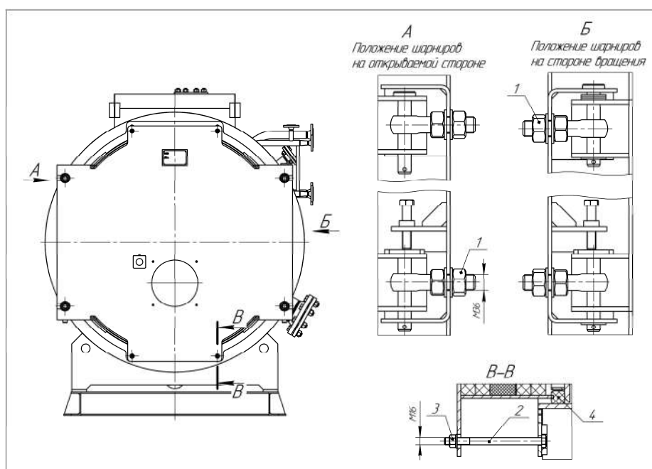
Рис. 21 Передняя крышка
